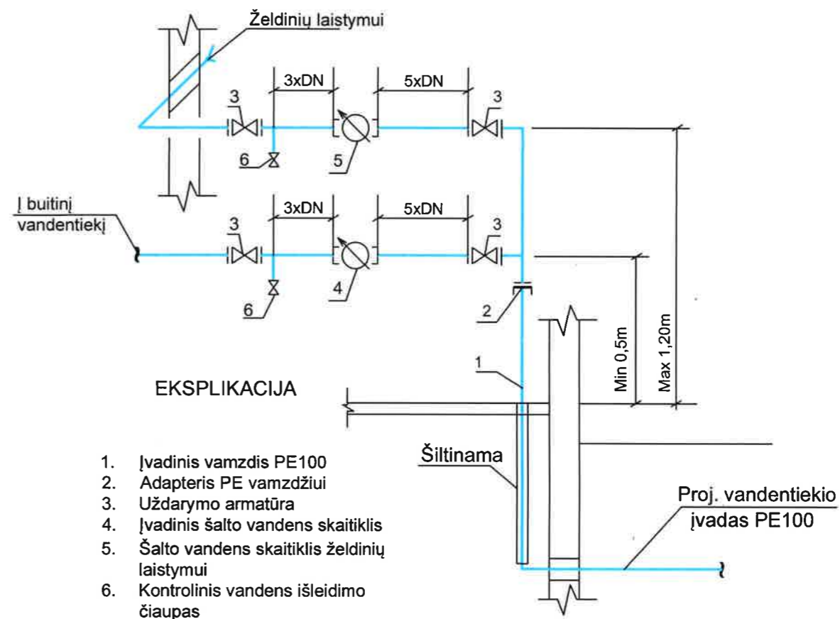
2 pav. Principinė VAM schema pastatui, kai projektuojama atšaka želdinių laistymui
