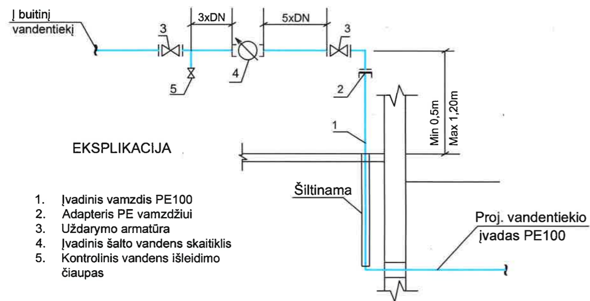
1 pav. Principinė VAM schema pastatui, kai pastate vanduo tiekiamas tik buitinėms reikmėms
